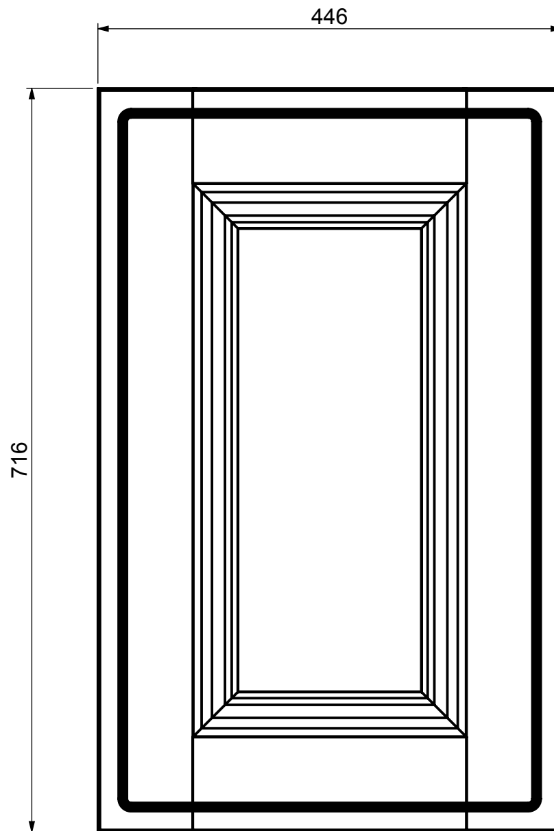
ANTA CON PANNELLO
