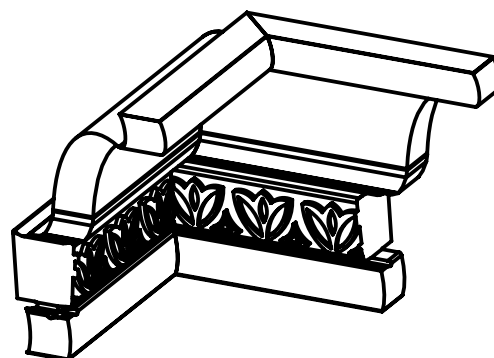
CAPITELLO INTERNO 90°
